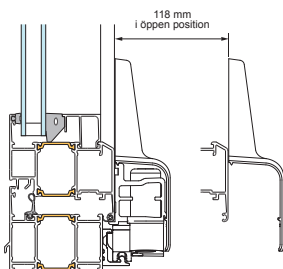
Underkant skjutfönsterdörr med beslag
