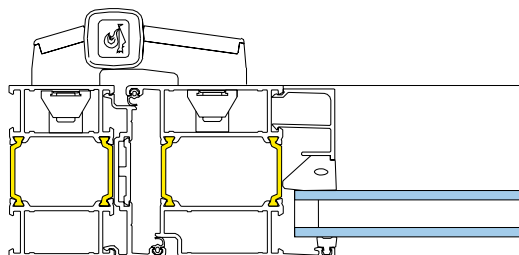
Karm med anslagsgående dörrblad
