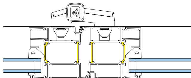
Viktörr, gångjärn insida
