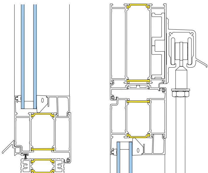
UK viktörr anslag mot tröskel. Alternativa trösklar finns.
