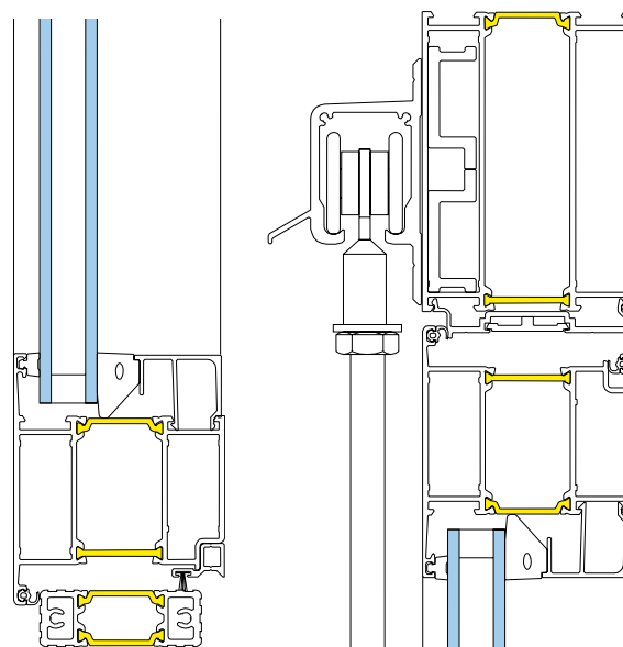
UK viktörr anslag mot tröskel. Alternativa trösklar finns.
