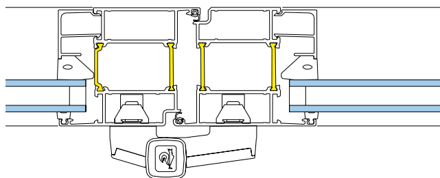
Viktörr, gångjärn utsida
