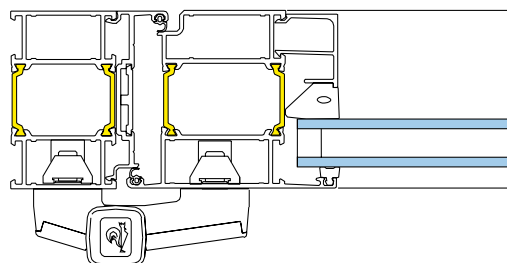
Karm med anslagsgående dörrblad
