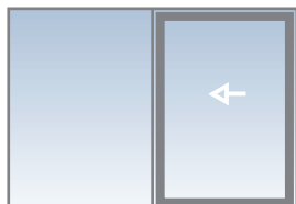
Enkelflyglig Fri öppning = karmyttermått/2 - 192 mm
