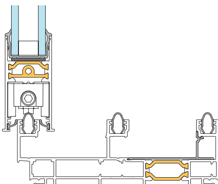
Trespårig med tre skjutbara dörrblad
