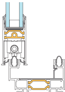
Tvåspårig med två skjutbara dörrblad
