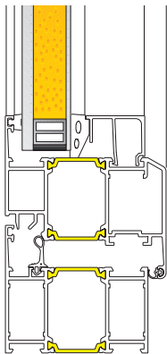
Båge, fyllning med Vaku Paneel
