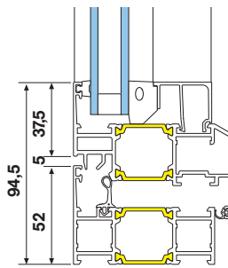
Karm/mellanbåge
