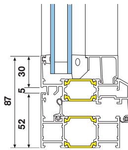
Karm/liten båge
