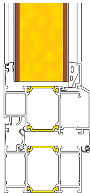
Båge med fyllning
