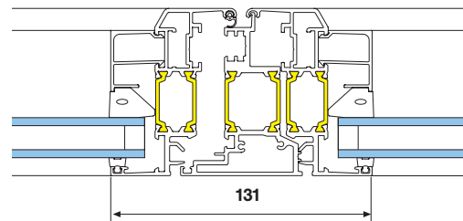
Mötesfönster utan mittpost
