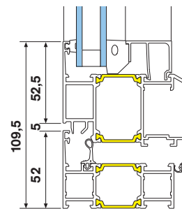
Karm/stor båge Båge till fönsterdörr
